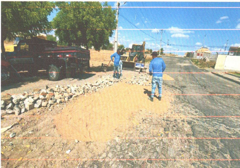
RECOMPOSIÇÃO DA PAVIMENTAÇÃO
