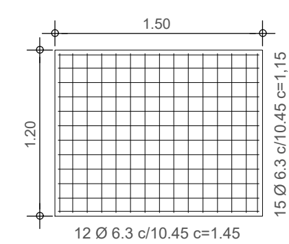
DETALHE DA ARMAÇÃO DA BOCA DE CONCRETO
