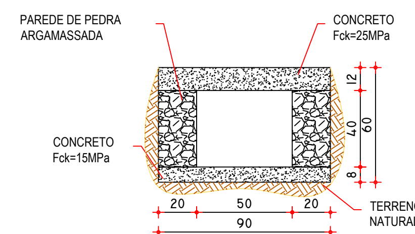
SEÇÃO TRANSVERSAL GALERIA - RAMAIS
