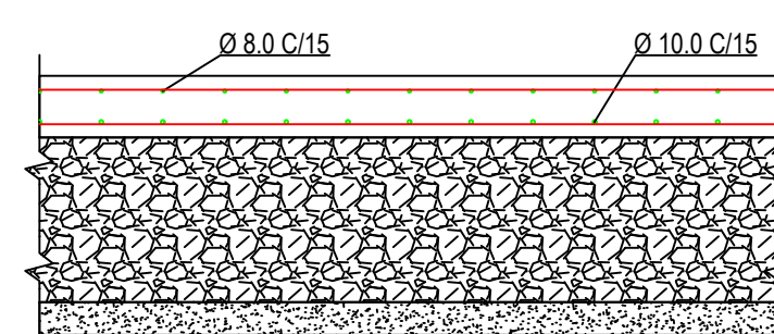
SEÇÃO LONGITUDINAL GALERIA - TRECHOS
