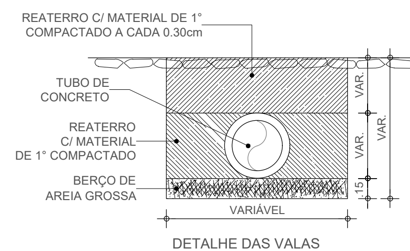
DETALHE DAS VALAS
