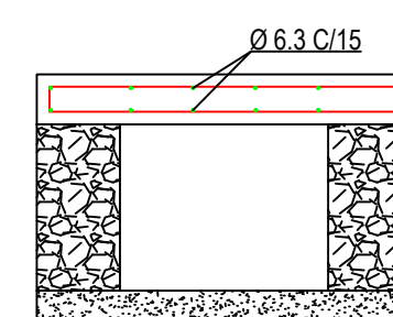
SEÇÃO TRANSVERSAL GALERIA - RAMAIS
