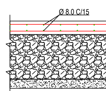
SEÇÃO LONGITUDINAL GALERIA - RAMAIS
