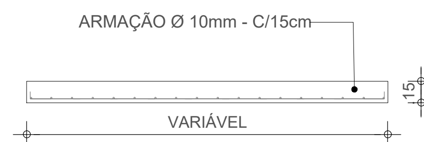
DETALHE LAJE SUPERIOR
