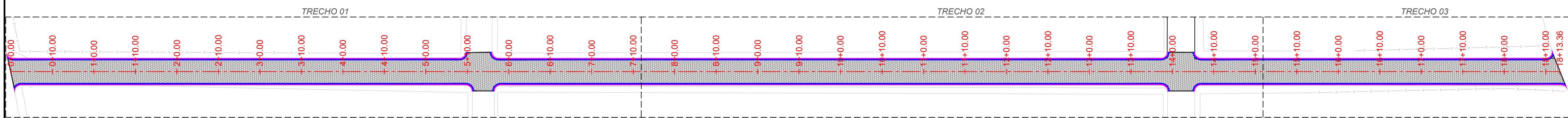
01 PLANTA RUA MARIA CLEMENTINA PINHEIRO - TRECHOS ESCALA 1 / 600
