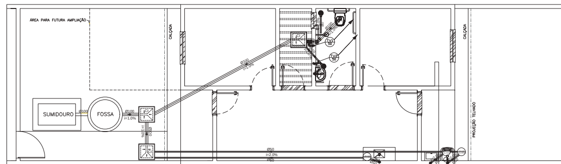
01 PROJETO SANITÁRIO ESCALA: 1:100
