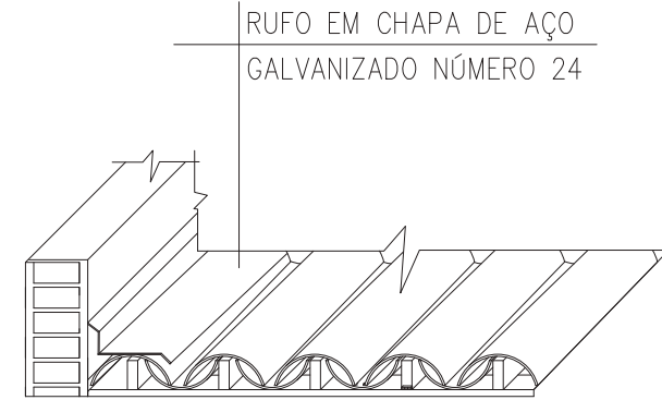
05 DETALHE RUFO ESQ. ESCALA
