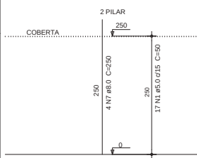
03 DETALHE DOS PILARES SEM ESCALA
