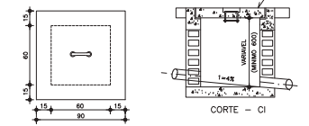
CORTE - CI
