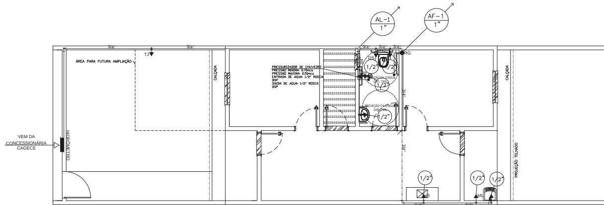
01 PROJETO HIDRÁULICO ESCALA: 1:100
