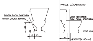
-DETALHE BACIA SANITARIA COM CAIXA ACOPLADA - DUCHA MANUAL
