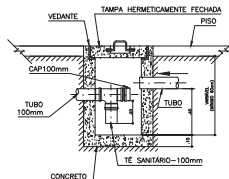
CORTE A-A
