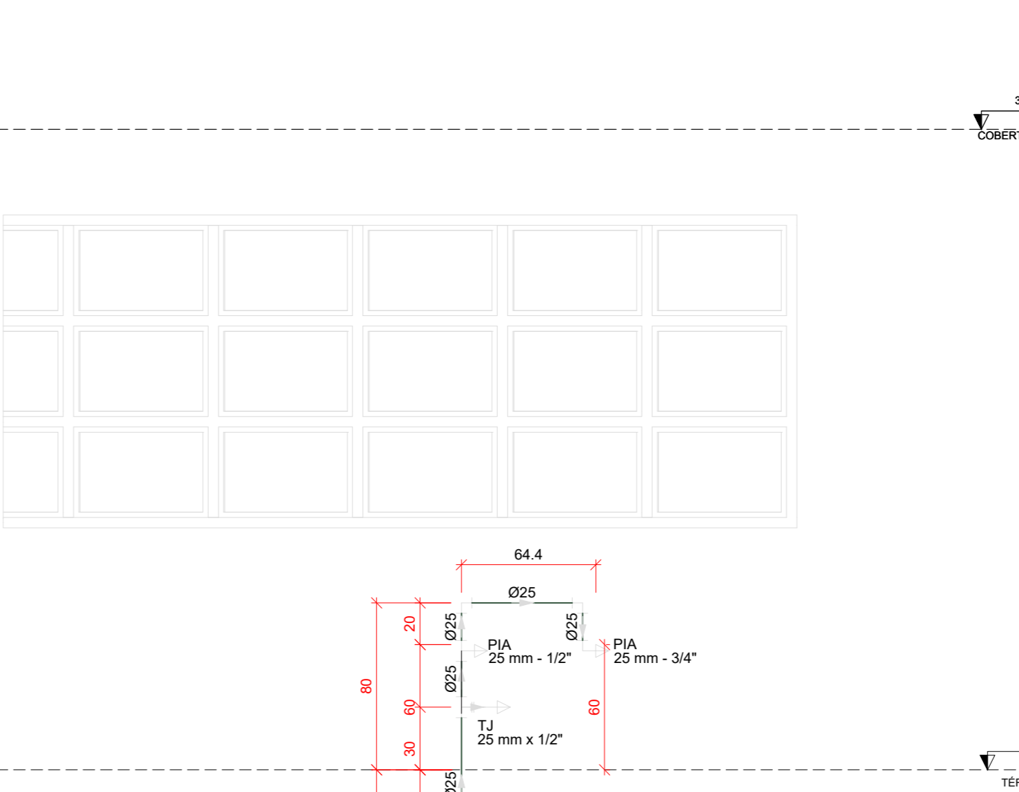
H48 DETALHE H48 ESCALA 1/25
