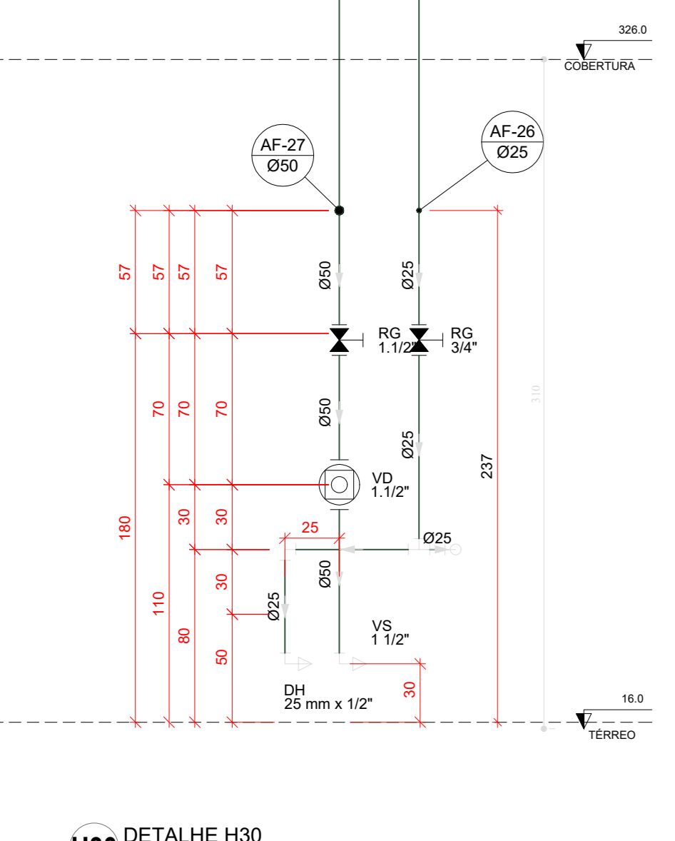
H31 DETALHE H31 ESCALA 1:25
