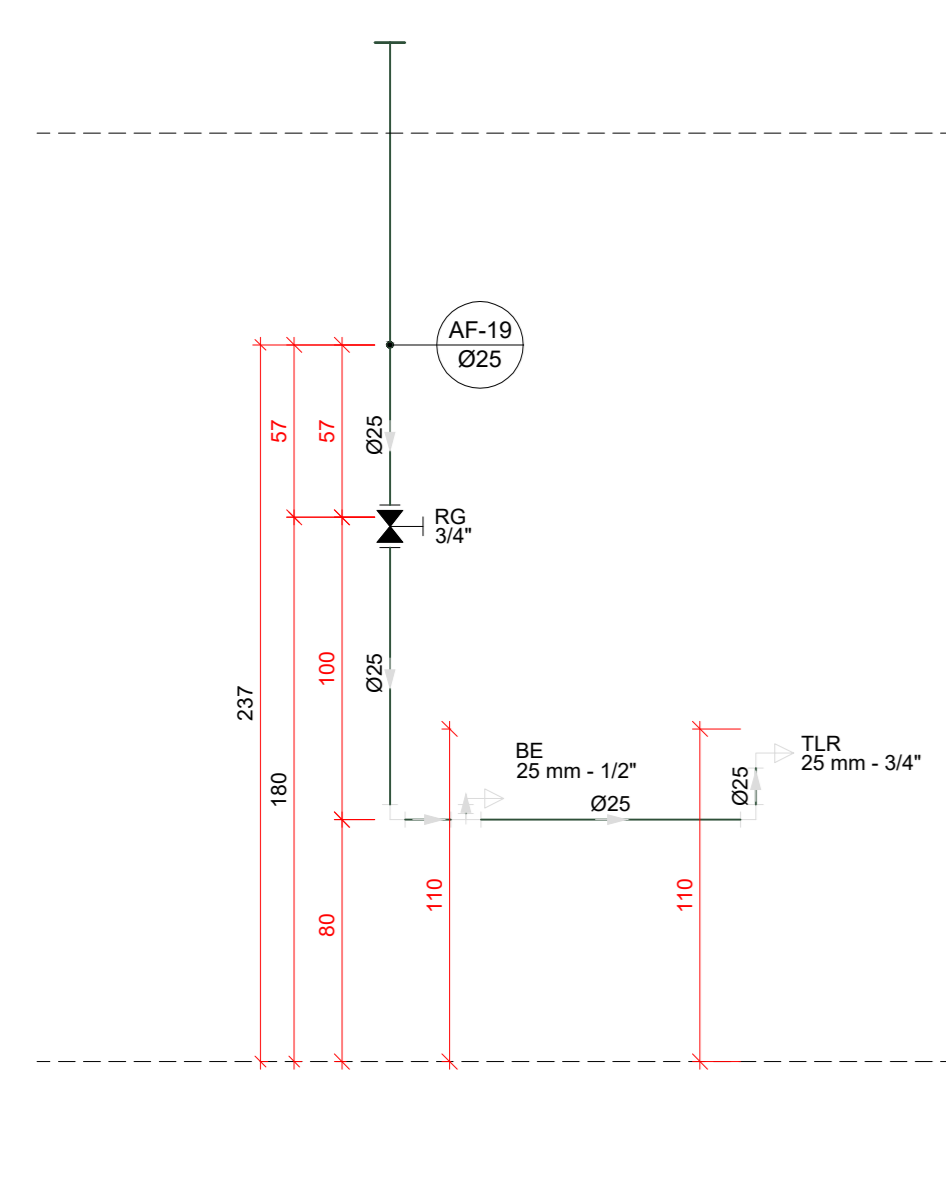
H21 DETALHE H21 ESCALA 1:25
