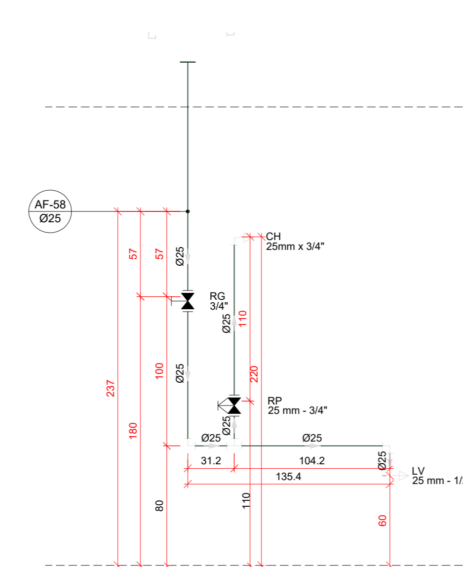
H46 DETALHE H46 ESCALA 1/25
