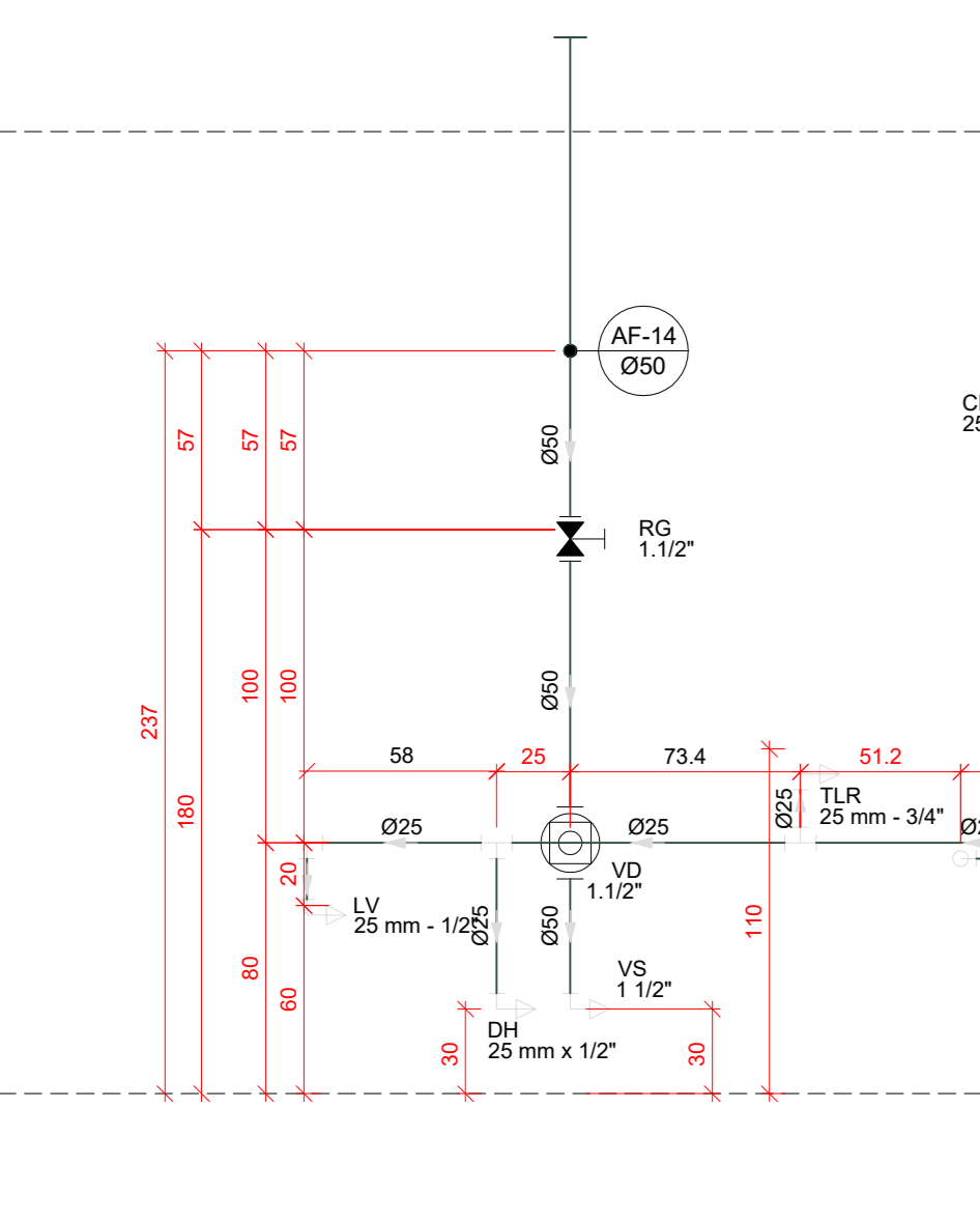
H26 DETALHE H26 ESCALA 1:25
