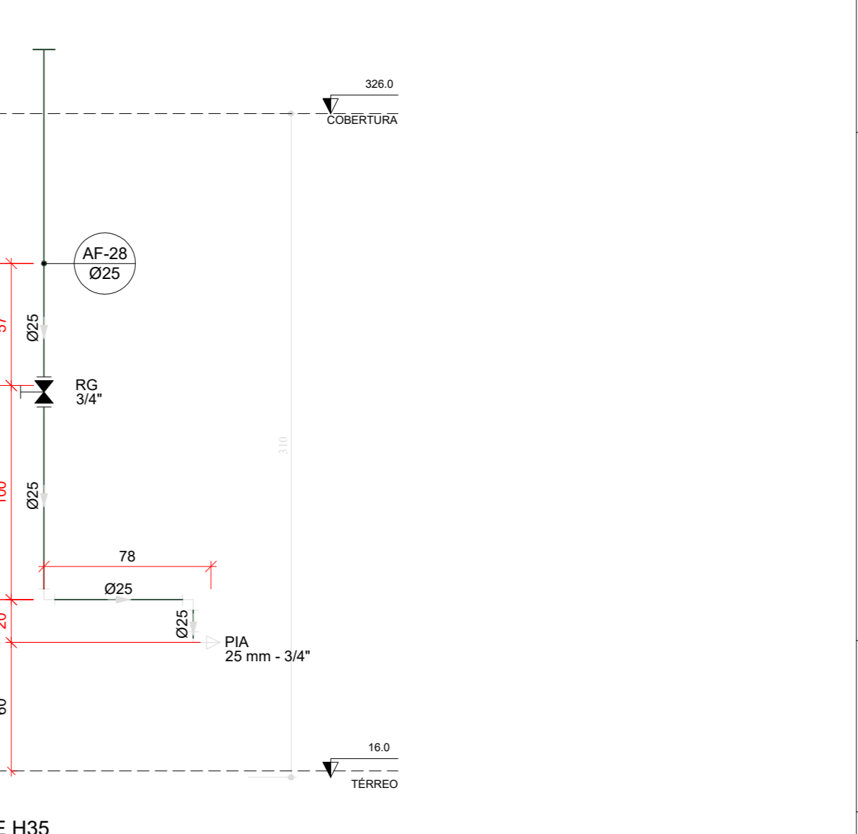
H35 DETALHE H35 ESCALA 1:25
