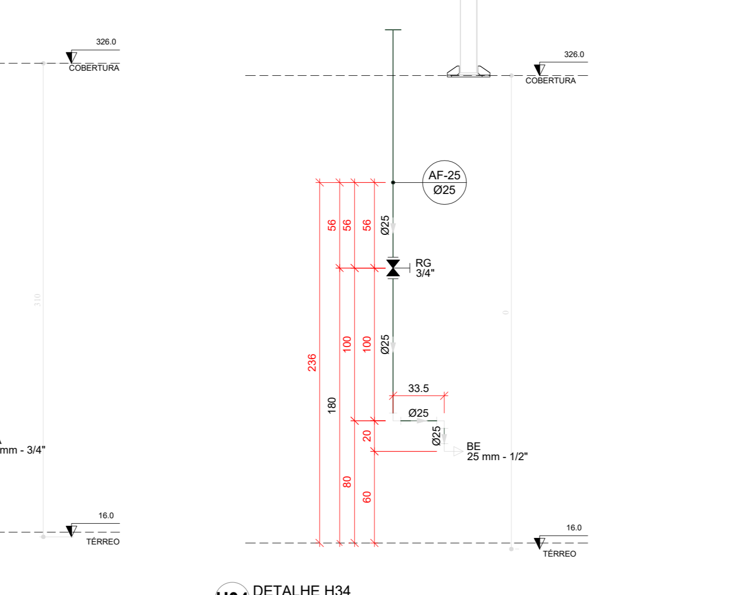
H34 DETALHE H34 ESCALA 1:25
