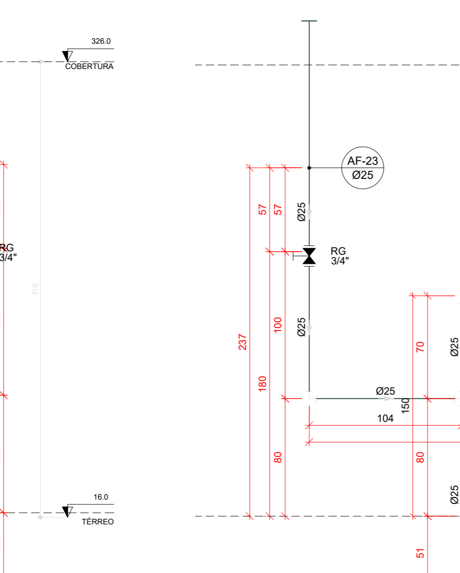
H27 DETALHE H27 ESCALA 1:25
