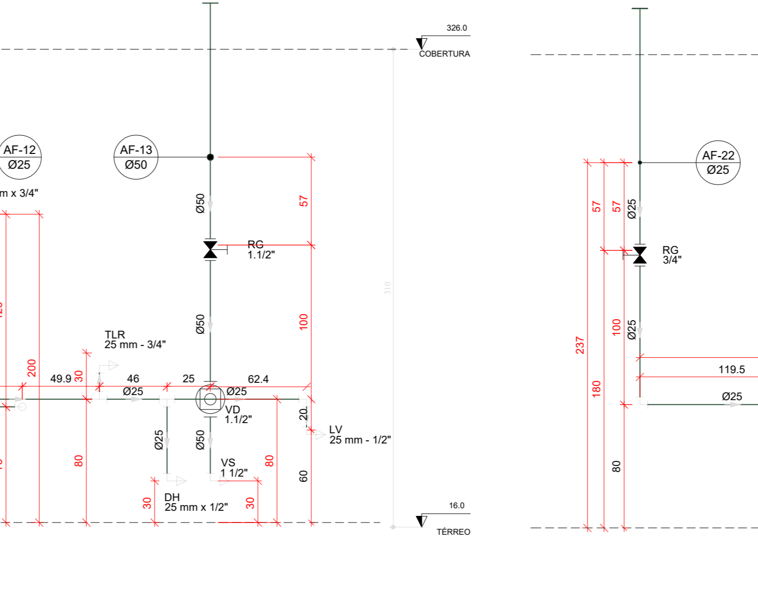
H24 DETALHE H24 ESCALA 1:25
