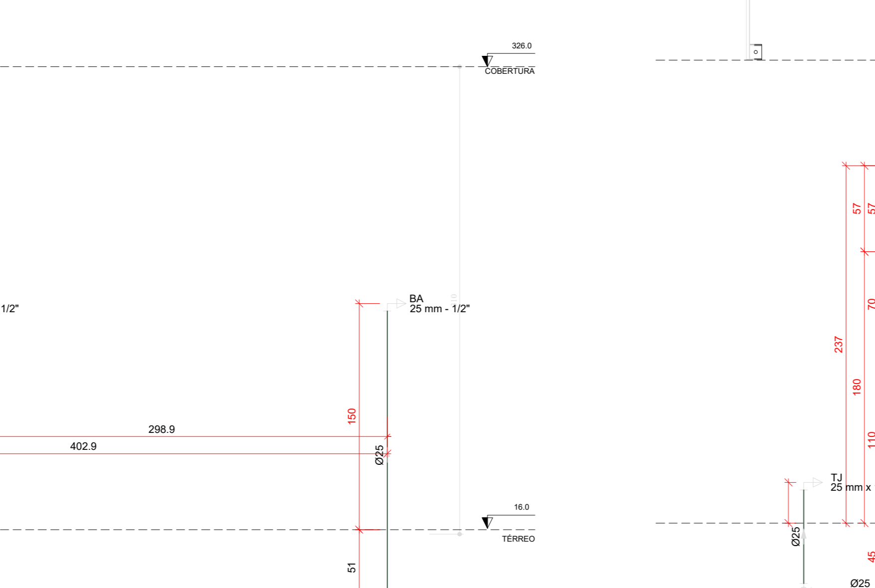
H28 DETALHE H28 ESCALA 1:25
