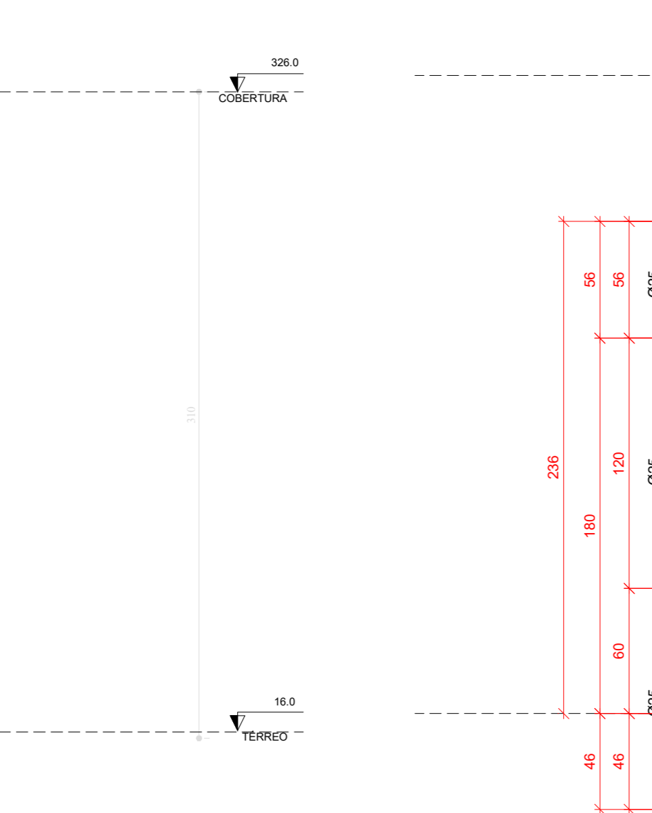
H22 DETALHE H22 ESCALA 1:25
