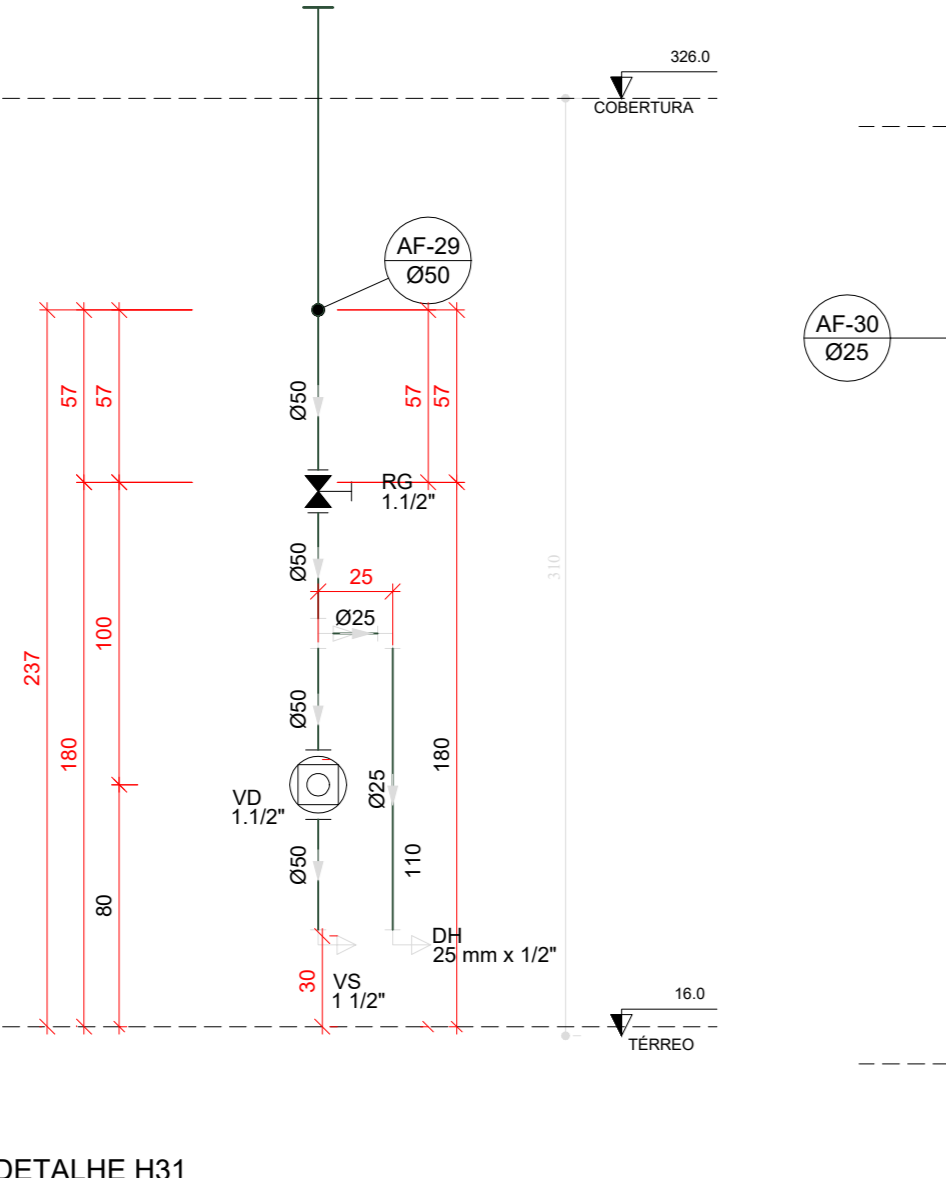
H32 DETALHE H32 ESCALA 1:25
